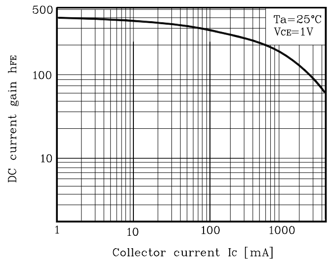
Fig. 4 h_{FE} - I_C
