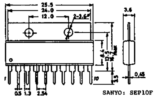
外形図 301BA-S10FIC (unit: mm)
