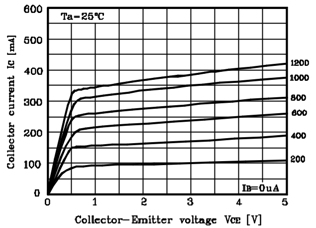
Fig. 4 I_C - V_{CE}
