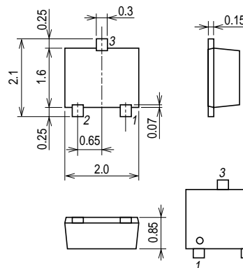
外形図 2167A
