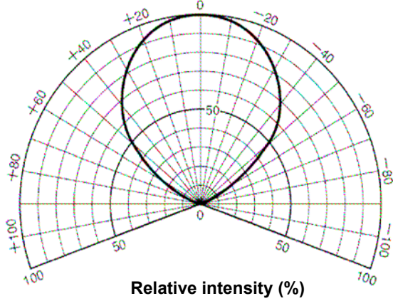
Radiant Pattern T_a=25^\circ C
