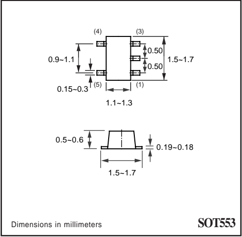
SOT553
