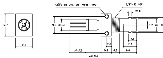
ST Receptacle
