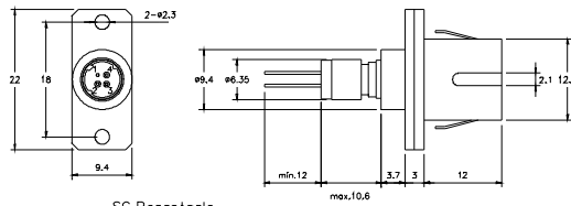
SC Receptacle
