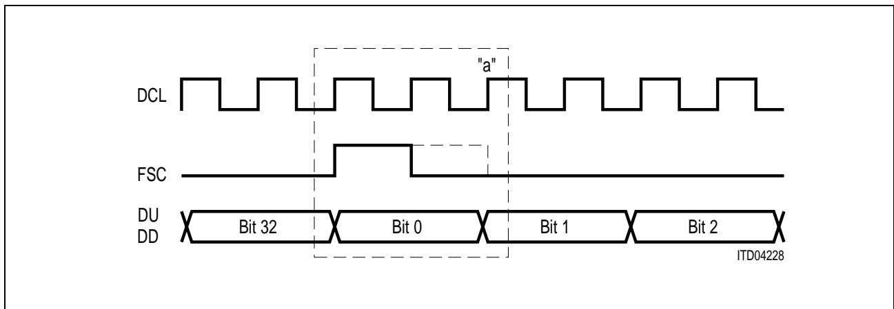
Figure 47 IOM ® -2 Interface Timing
