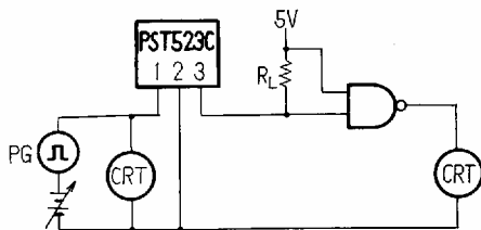
R L : 4.7k TTL IC Combination
