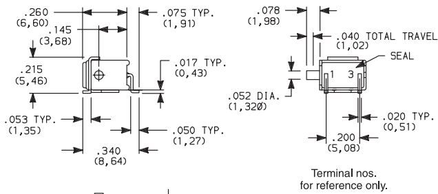
GP11- omit hole 2.
