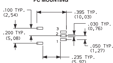
GP11- omit pad 2.
