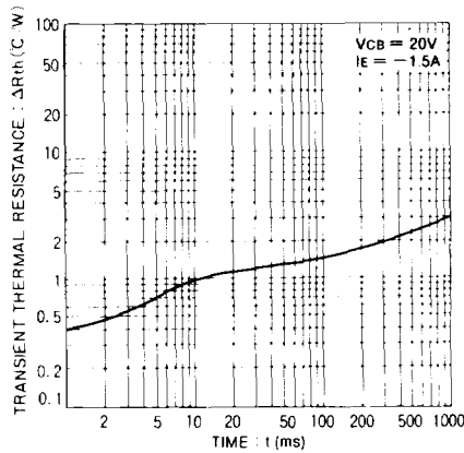
Fig.3 過渡熱抵抗
