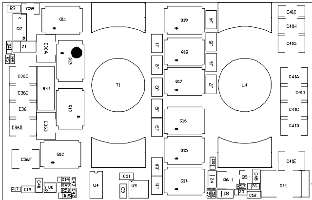
The hottest component on the top side: Q13
