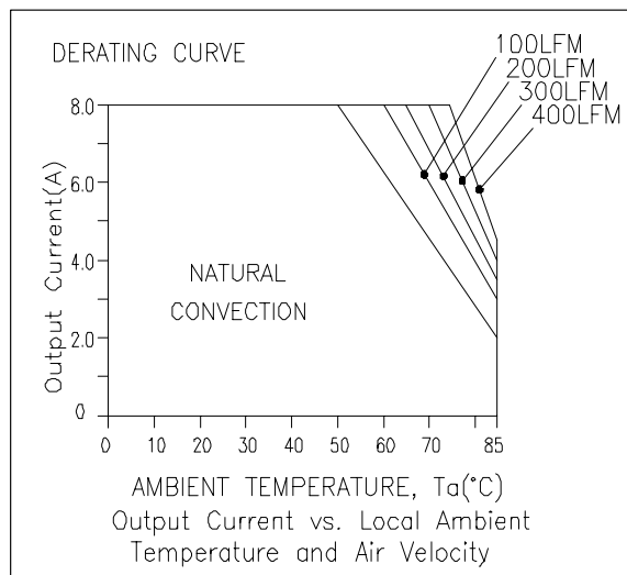
Vo=3.3V
