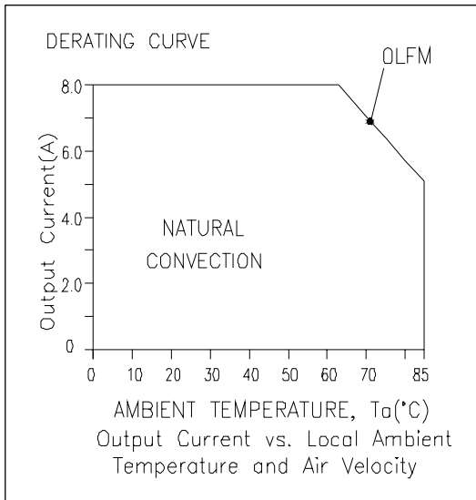
Vo=0.9V
