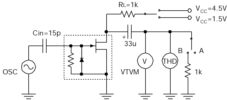
Specified Test Circuit
