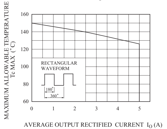
T_c - I_O
