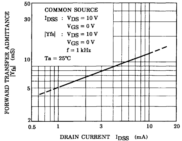
|Yfs| - IDSS
