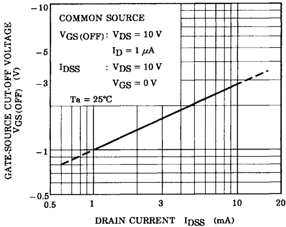
VGS(OFF) - IDSS
