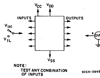
Fig. 8 - Input voltage.
