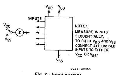
Fig. 7 - Input current.
