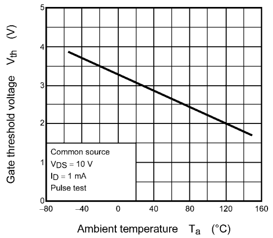
Fig. 8.10 V th - T a
