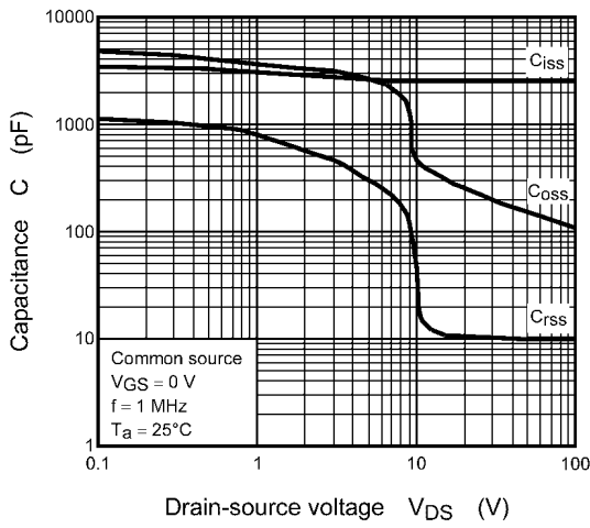
Fig. 8.9 C - V DS
