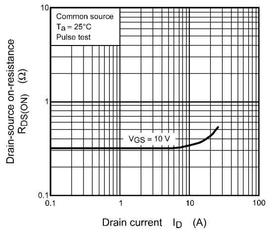
Fig. 8.6 R_{DS(ON)} - I_D
