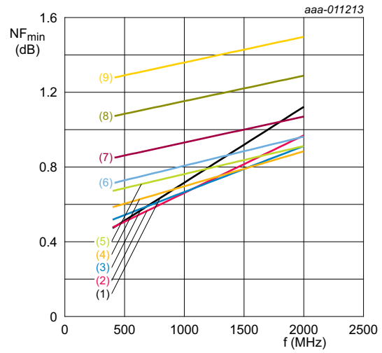
V CE = 8 V; T amb = 25 °C; Γ S = Γ opt . (1) I C = 1 mA (2) I C = 2 mA (3) I C = 3 mA (4) I C = 5 mA (5) I C = 8 mA (6) I C = 10 mA (7) I C = 15 mA (8) I C = 25 mA (9) I C = 35 mA
