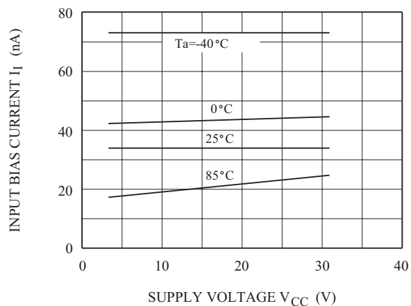
V_{CC} - I_I
