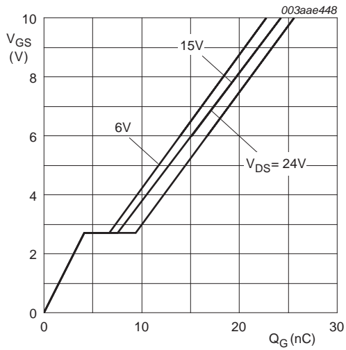
T_j = 25^\circ\text{C}; I_D = 15\text{A}
