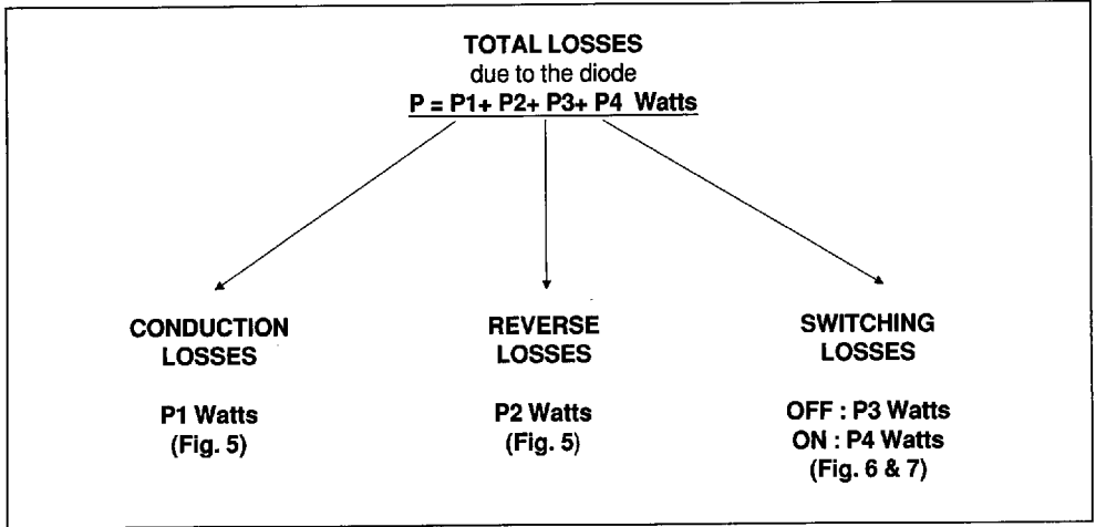
Fig. 2 : CLAMPING DIODE.
