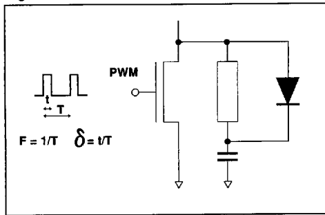
Fig. 3 : DEMAGNETIZING DIODE.
